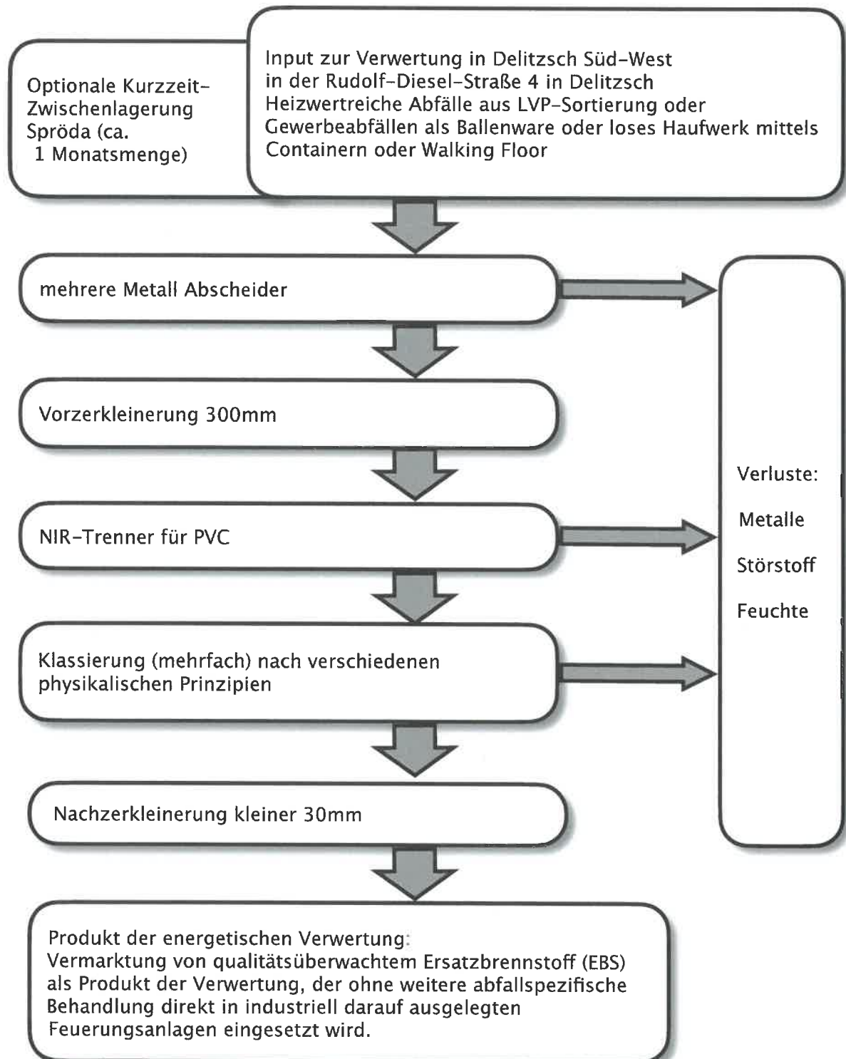
Bild 1: Fließbild der energetischen Verwertung Kreiswerke Delitzsch GmbH in Delitzsch
